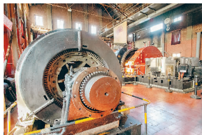
开滦唐山矿的1号绞车于20世纪三十年代建成，通过牵引升降机完成人、物运输。由于仍在运转，现场不能展示其内部结构。而在网上则可以通过建模和虚拟运转来说明其功能和原理。
