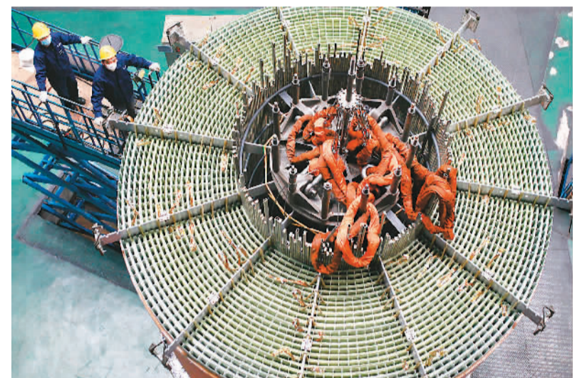
武汉西北城区供电电源点某重要变电站近日因设备故障造成电网补偿能力下降。中国能建北京电力设备总厂有限公司迅速行动，加班加点完成3台替换设备的生产和包装，当日启程发往武汉。图为2月28日，工人正在对电抗器进行最后检查。 本报记者 贺勇摄
