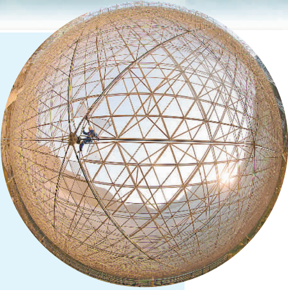
工作人员检修FAST反射面板。（新华社发）
