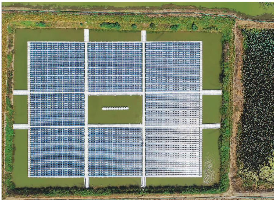
图为在安徽省天长市秦栏镇牧马湖养殖水域漂浮式光伏发电站，电力工人在对发电设备进行巡视检查（无人机拍摄）。
