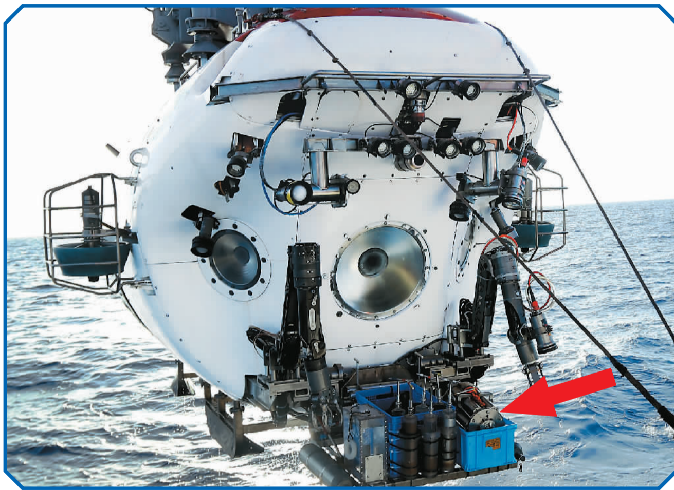
5月25日，“蛟龙”号载人潜水器在马里亚纳海沟成功找到一年前因特殊情况留在了6300米大洋深处的采水器，“大海捞针”的故事变为现实。图为刚从深海归来的“蛟龙”号。其最右边样品筐内的物品，即成功回收的Gas-tight采水器(气密性耐压序列采水器)。
