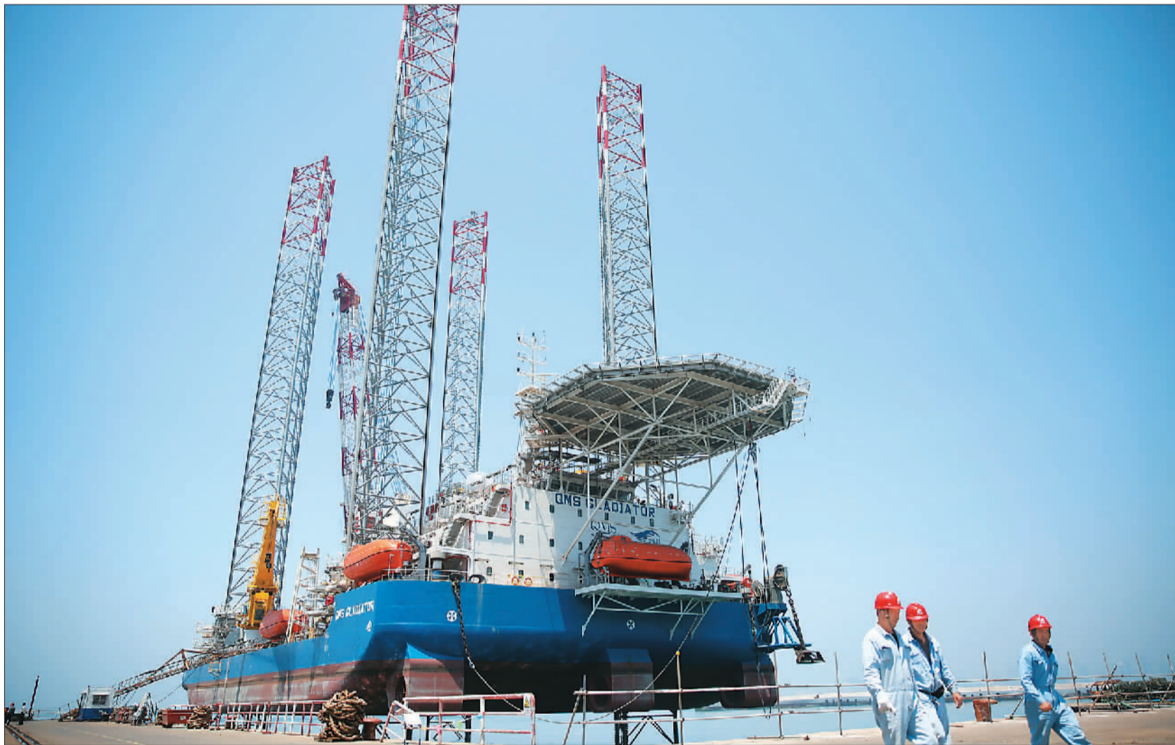
5月24日，在青岛海关关员的监管下，中国首个110米桁架式自升式海工平台（阿布扎比SE—350LB海工平台）从青岛海西重工有限责任公司码头顺利发运，出口目的地为中东国家阿联酋。该平台可用于海上修井、采油、风电安装、起重等辅助作业。图为工人从在建的第三台110米桁架式自升式海工平台前走过。张进刚 郑长江摄影报道（人民视觉）
