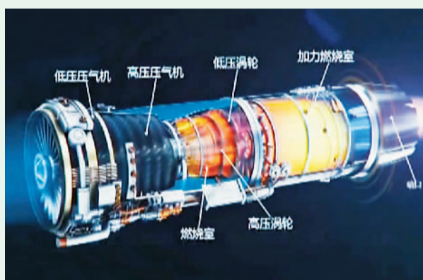
航天发动机示意图(资料图片)
