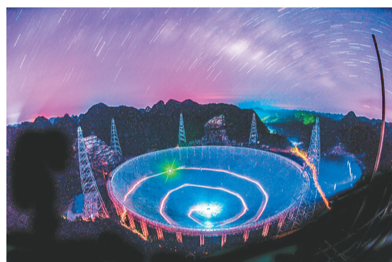
2016年6月27日，贵州省黔南布依族苗族自治州平塘县，星空下的500米口径球面射电望远镜。欧东衢摄
