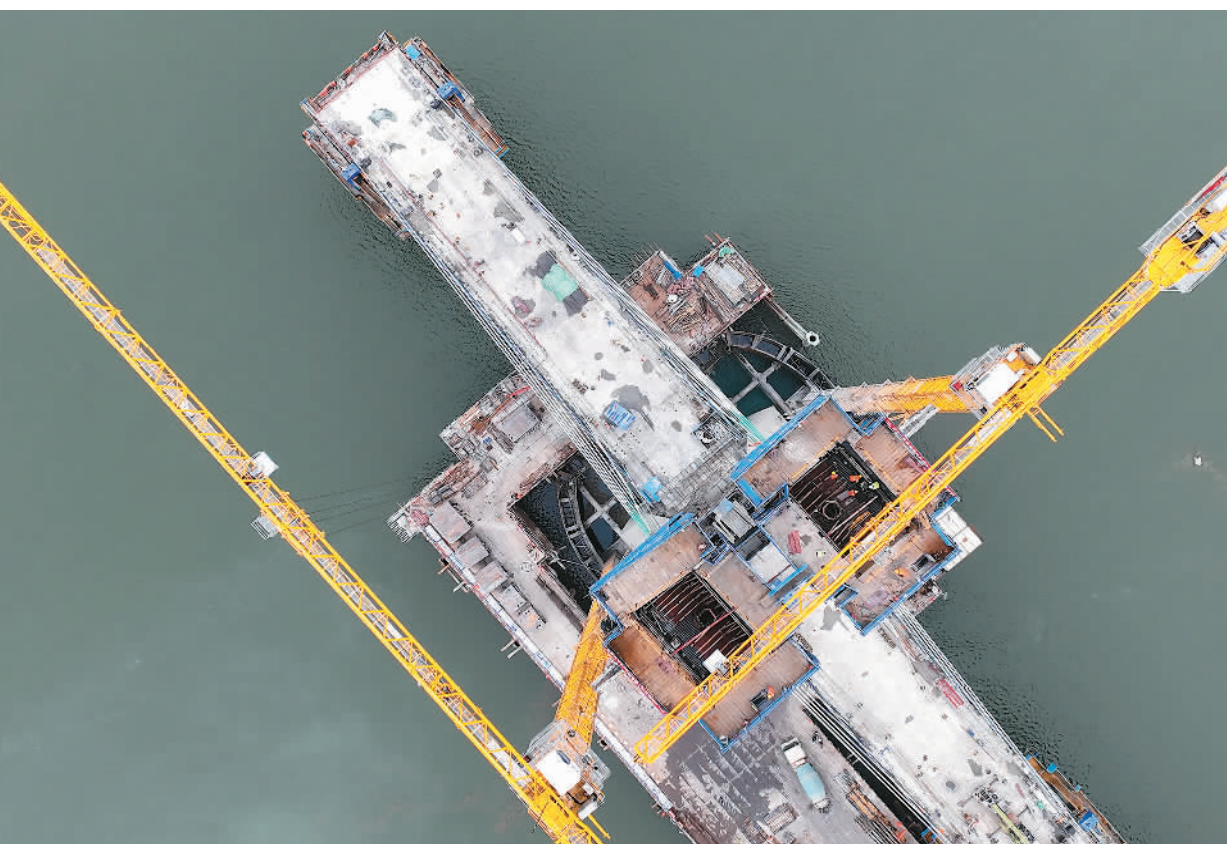
4月16日，由中铁十一局承建的沪渝蓉高铁武宜段钟祥汉江特大桥316号主塔顺利封顶，标志着这座高速铁路无砟轨道混凝土梁斜拉桥两座主塔全部封顶。沪渝蓉高铁是中国“八纵八横”高铁网沿江高铁通道的重要组成部分，其中，武汉至宜昌段正线全长313公里。钟祥汉江特大桥横跨汉江，是沪渝蓉高铁武宜段的关键控制性工程。图为4月16日拍摄的沪渝蓉高铁武宜段钟祥汉江特大桥316号主塔施工现场。新华社记者 杜子璇摄
