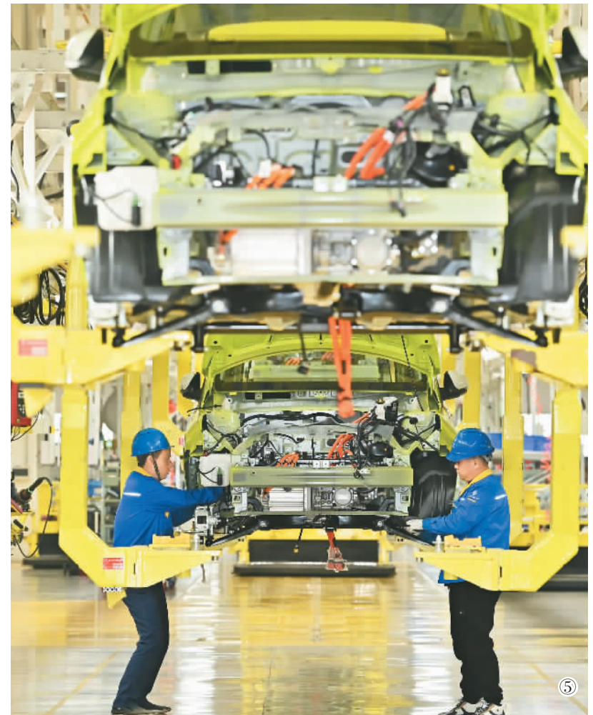
图⑤：江西一家新能源汽车有限公司总装车间生产线上，工人正在加紧生产赶订单。
