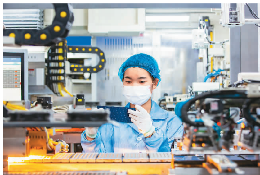
江苏省海安市整合当地光伏产业资源，实施自动化、信息化、智能化升级改造，持续提高光伏产业竞争力。图为海安市一公司车间内，工人们正在赶制出口太阳能光伏组件。 翟慧勇摄（人民视觉）
