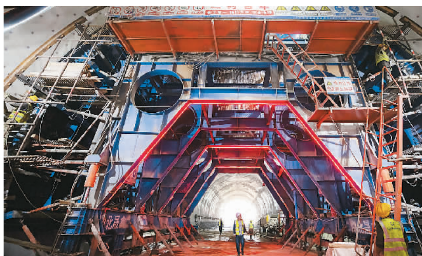
近日由中铁七局承建的新建沪渝蓉高铁武宜段7标罗家村隧道顺利贯通，成为全线首座贯通的隧道。据悉，新建沪渝蓉高铁是国家“八纵八横”高铁骨干通道之一，建成后东西横贯国内6个省份，串联起长三角城市群、长江中游城市群和成渝双城经济圈，对构建长江综合交通运输体系和推进长江经济带发展具有重大意义。图为建设现场。 郭强摄
