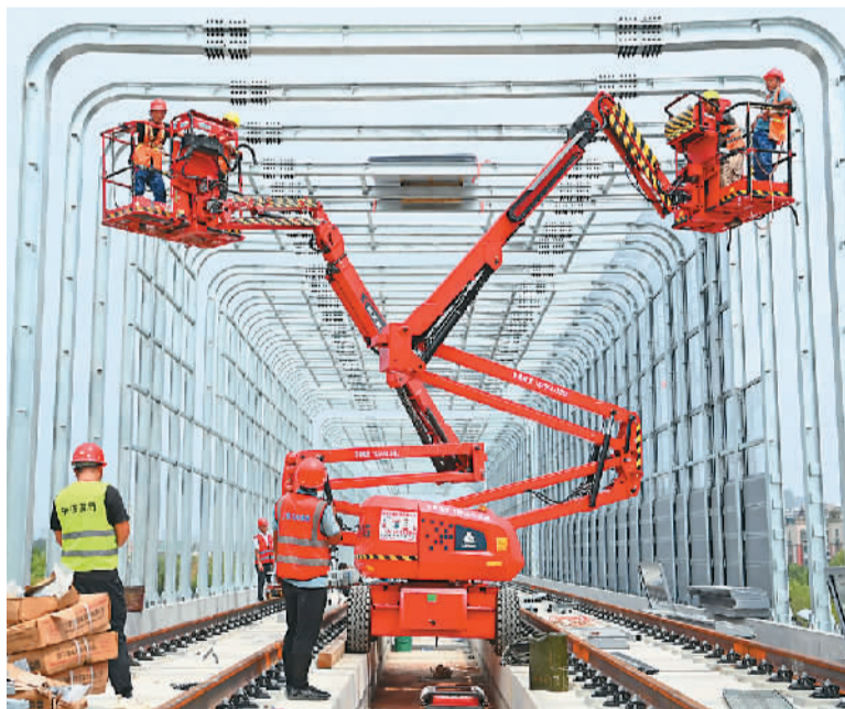
中秋假期，铁路建设者坚守岗位，推进建设，确保进度。图为在安徽省滁州市南谿区腰铺镇，建设者在滁(滁州)宁(南京)城际铁路二期高架线上安装环保声屏障。
