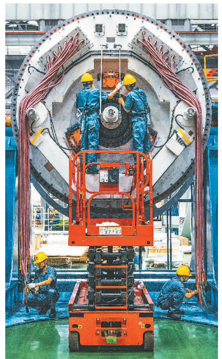
近日，在广东省阳江市明阳阳江智能制造中心风电整机装配车间里，工人通过吊机忙着对机舱和轮毂进行配件安装，开足马力赶订单。作为全球海上风电单体产能最大智能制造中心，该中心研发、制造的产品主要服务于沿海地区海上风电产业，畅销海内外市场。图为工人正在对产品进行配件安装调试。邱新生摄（人民视觉）
