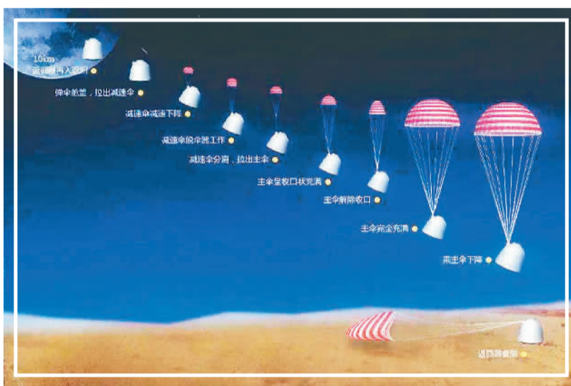
嫦娥五号返回器着陆过程示意图
