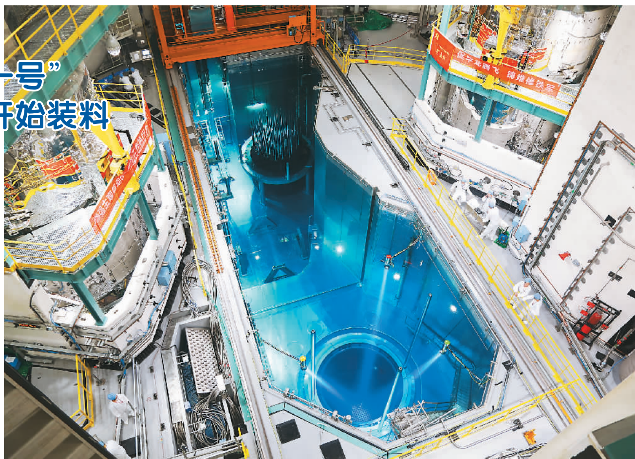
“华龙一号”全球首堆福清核电5号机组装料水池。
