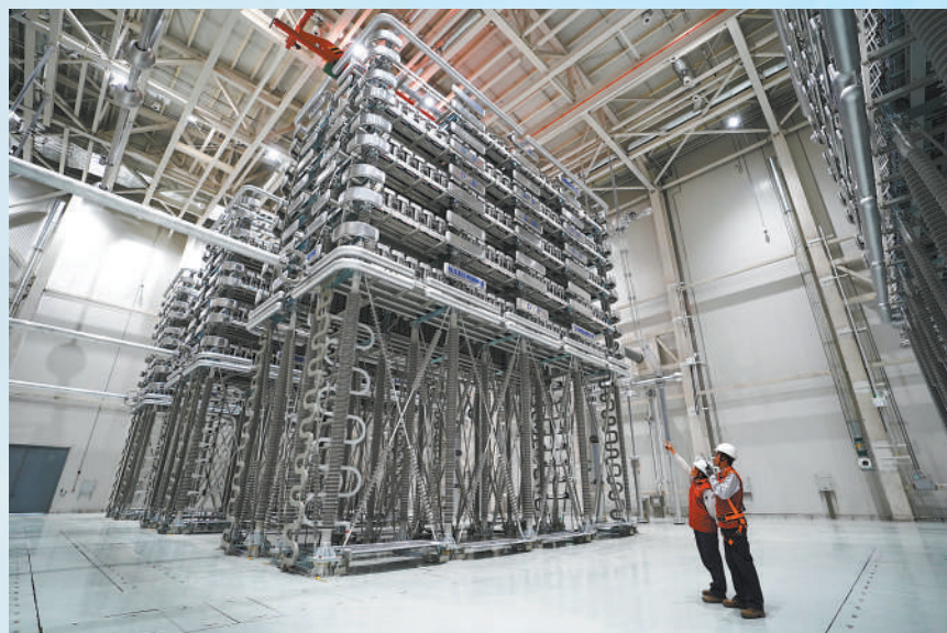
▲南瑞集团工程人员在白鹤滩—江苏±800千伏换流站内开展换流阀检修工作。杨铭轩摄(人民视觉)
