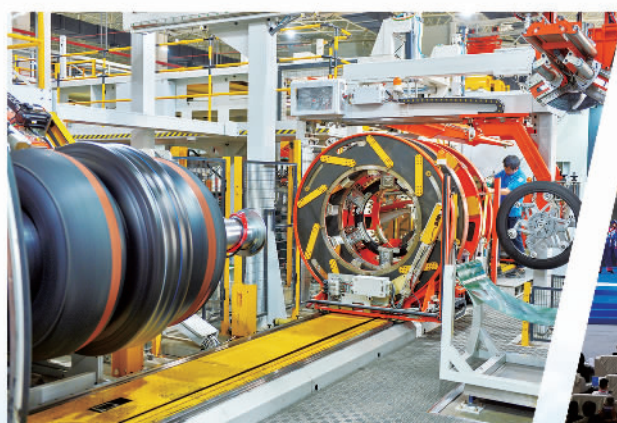
贵州持续推动产业升级。图为贵州轮胎股份有限公司全钢三期项目车间
