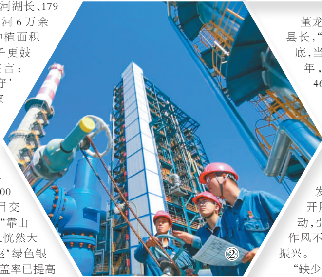
图②：大庆石化技术人员检查生产设备。
