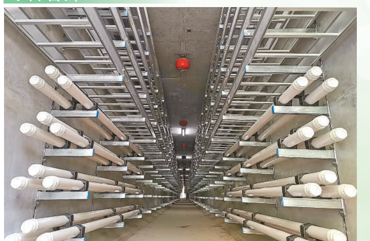
幸福林带综合管廊电力舱。 王 健 摄
