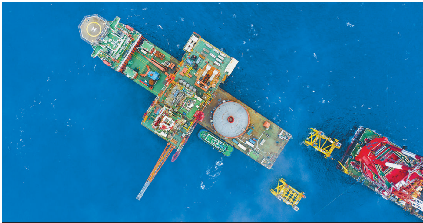
本报北京5月14日电（记者冉永平、丁怡婷）记者从中国海油获悉：13日，万吨级海上油气平台恩平20—4钻采平台在珠江口盆地海域完成安装，创造了我国海上油气平台动力定位浮托安装重量新纪录。
