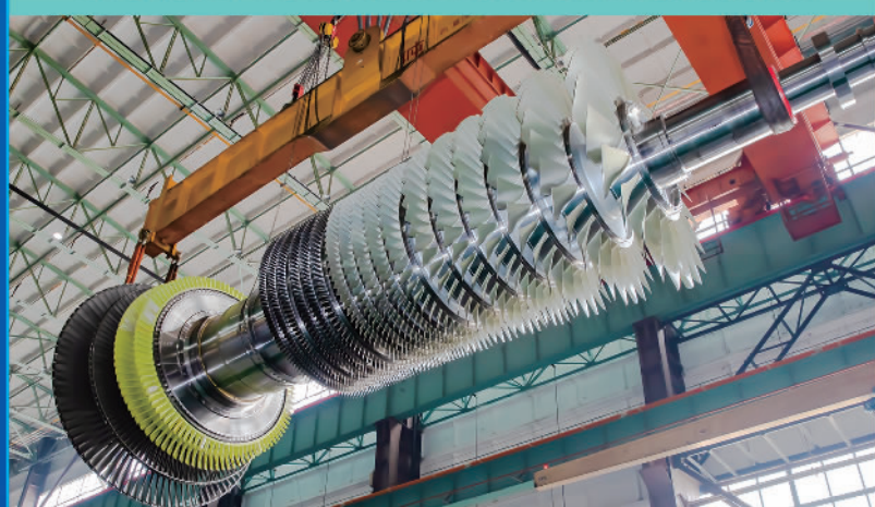
东方汽轮机有限公司制造的高国产化率重型燃气轮机转子
