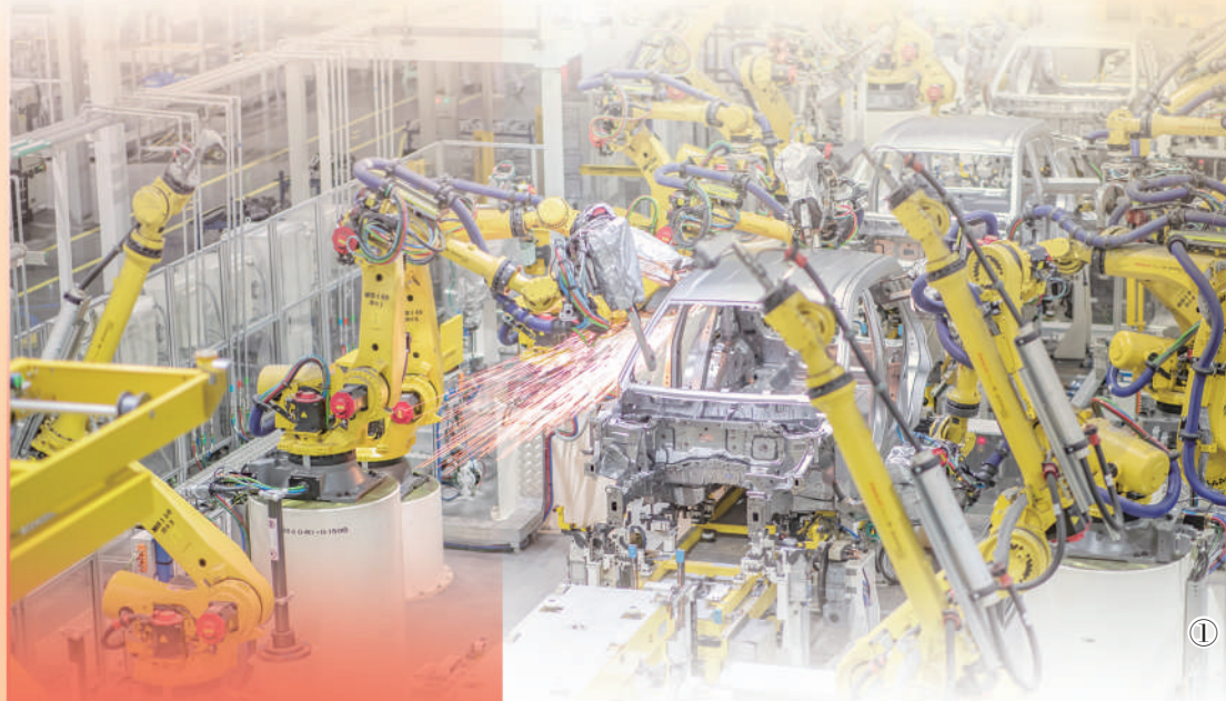
图①:在重庆一家智能工厂焊装车间,点焊机器人正在进行焊接作业。
