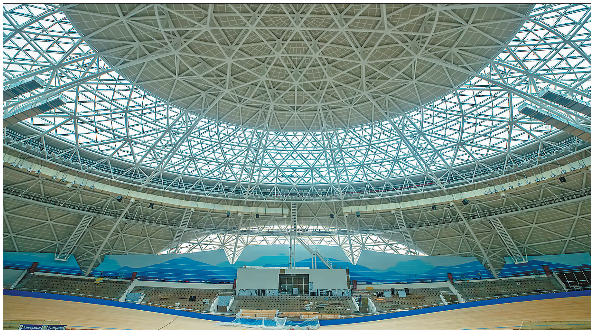
杭州亚运会淳安场地自行车馆即将竣工 位于浙江省杭州市淳安县界首乡的2022年杭州亚运会淳安场地自行车馆建设项目工程,日前进入收尾施工阶段,工作人员正在进行场内赛道、护栏和场外装饰、景观施工,全部工程预计将在4月底竣工。 毛勇锋摄(影像中国)
